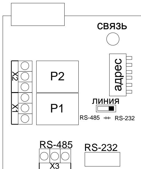
Рис. 1. Внешний вид платы
